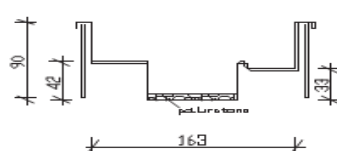
SEZIONE B-B
